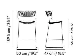
iSi 8261 Stool 65
