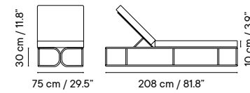
iSi 8194 Sunlounger
