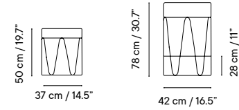
iSi 9160 Pouf
